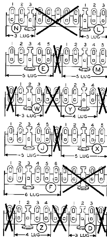
Detail 1A
