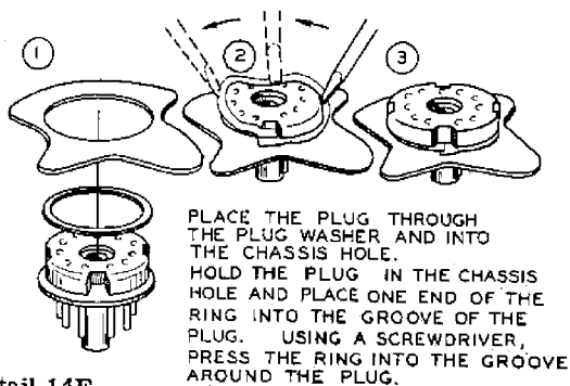
Detail 14E
