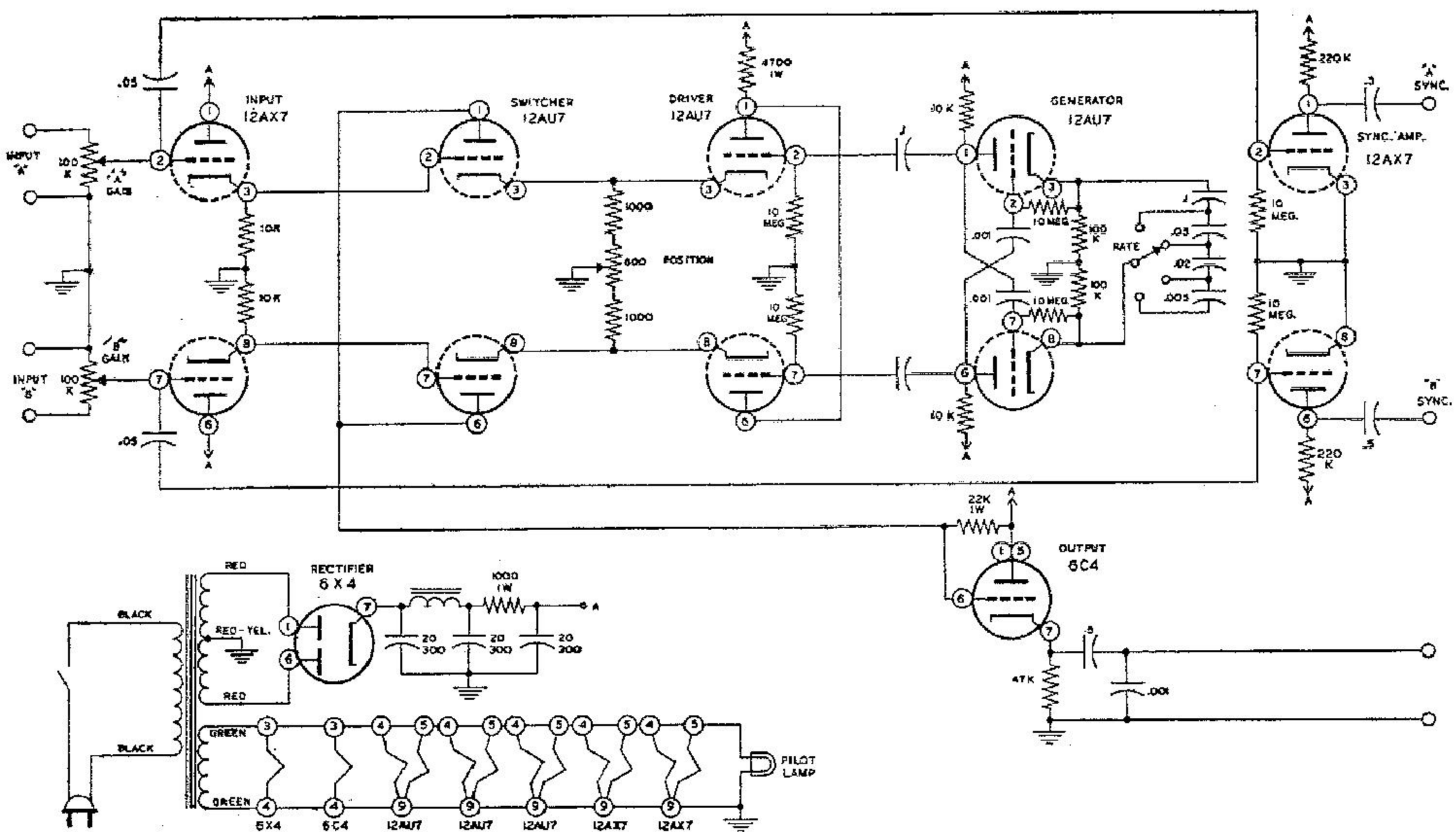
Schema del commutatore elettronico Heath S3.
