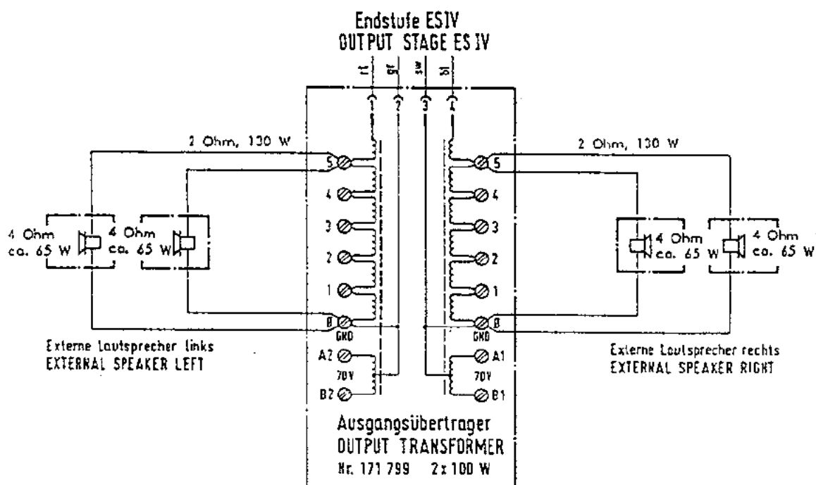
Anschluschema für Ausgangsübertrager CONNECTION DIAGRAM FOR OUTPUT TRANSFORMER
