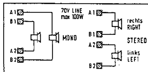
Anschluschema für Ausgangsübertrager CONNECTION DIAGRAM FOR OUTPUT TRANSFORMER
