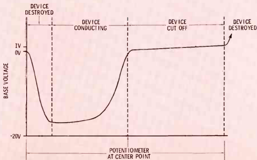
Fig. 9 Transistor base-voltage diagram.
