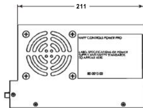
Tapped 6-32 (4)
