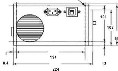
Tapped 6-32 (4)
